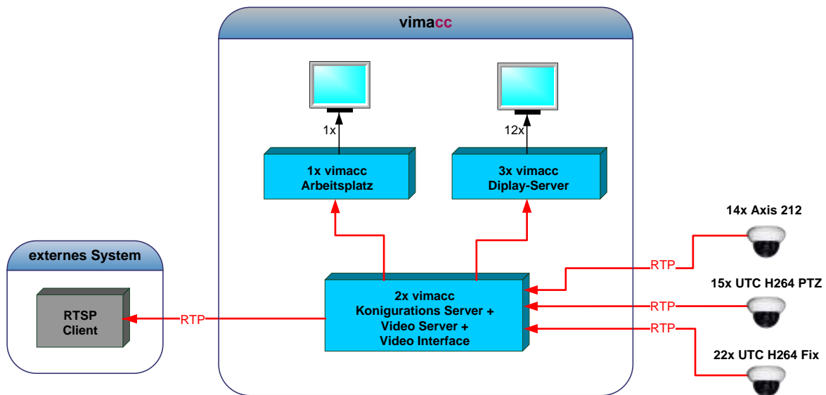
Abbildung 2.1: vimacc Referenzsystem
