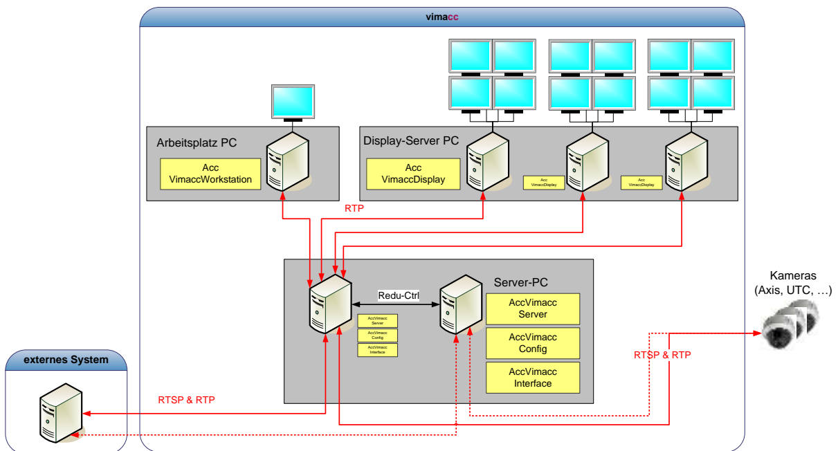
Abbildung 2.2: vimacc Referenzsystem - Prozessverteilung
